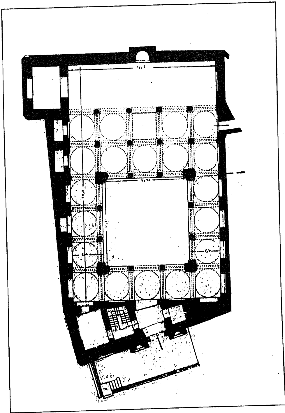
شكل (١٩) جامع الأقمير، مسقط أفقى عن أحمد فكرى.
